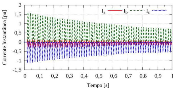
Figura 3 - Corrente nos terminais do lado de alta tensão na energização do autotransformador de 230/138/13,8 kV – 150 MVA (ATR) da SE J. Teixeira.
